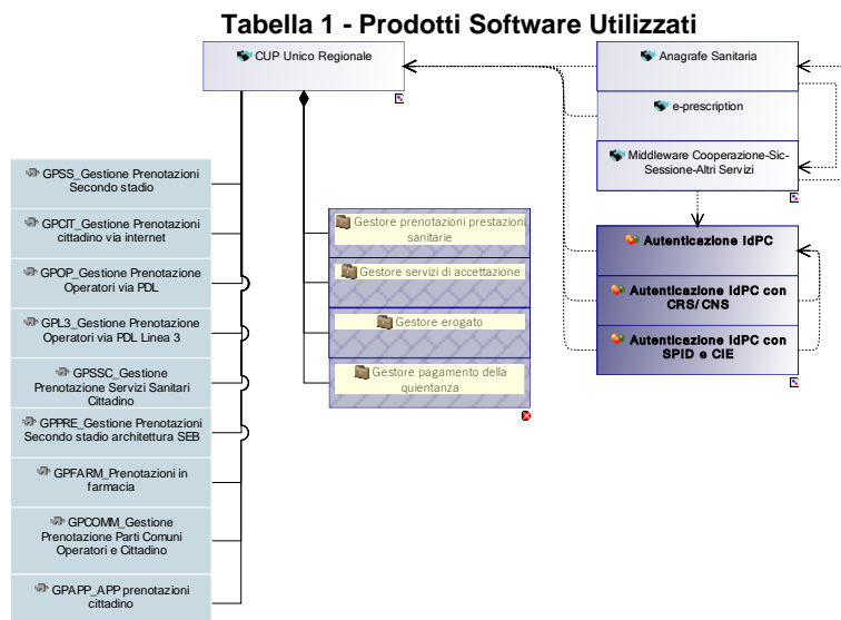
Figura 1 - Architettura del Servizio
